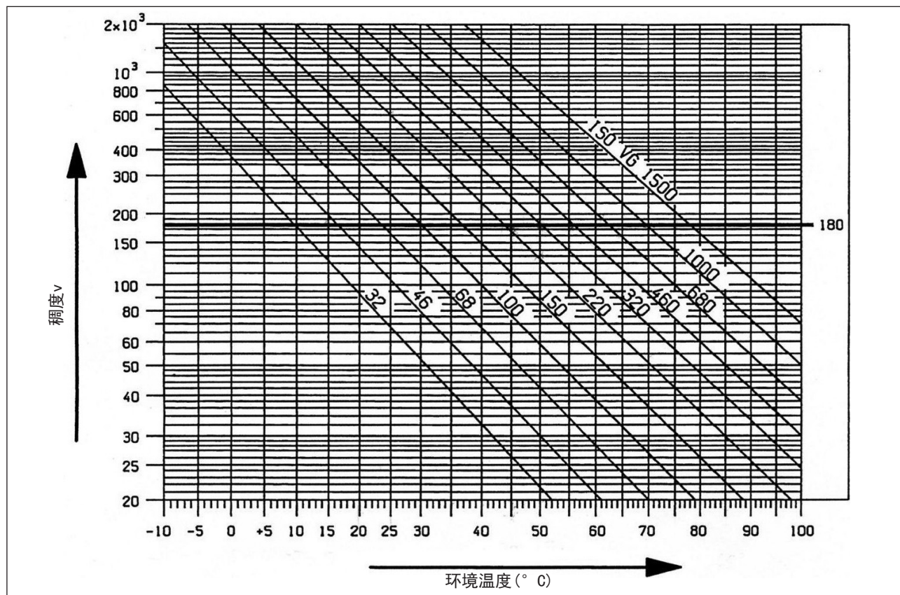
稠度/环境温度图表
