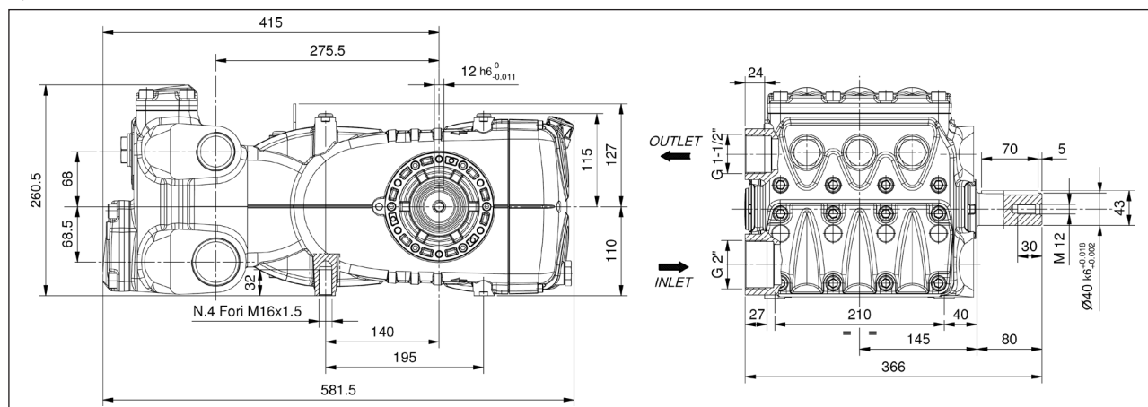
Сухой вес 75 кг
