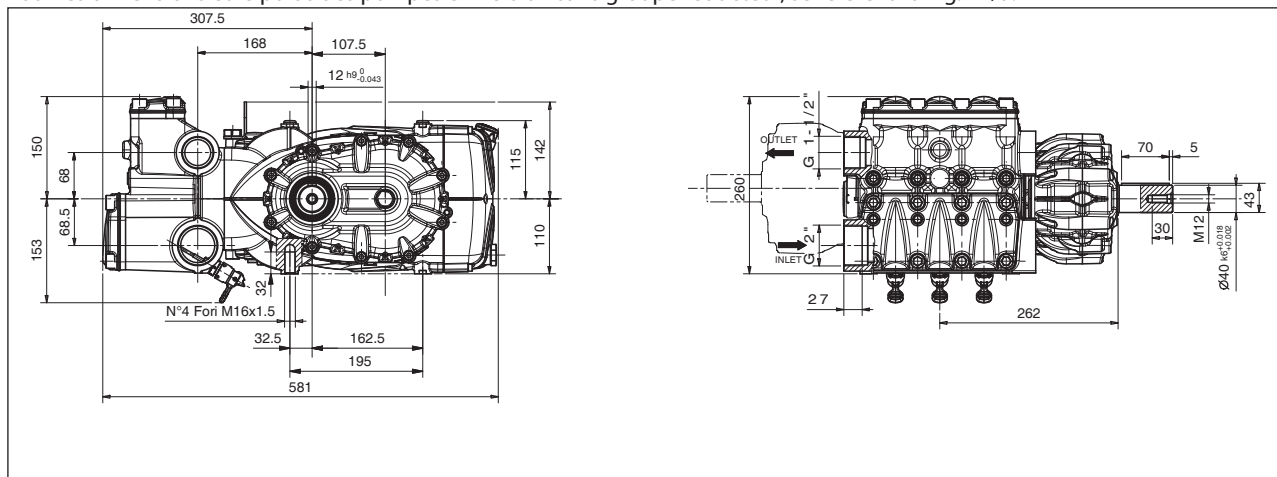
Poids à vide 80 kg.
