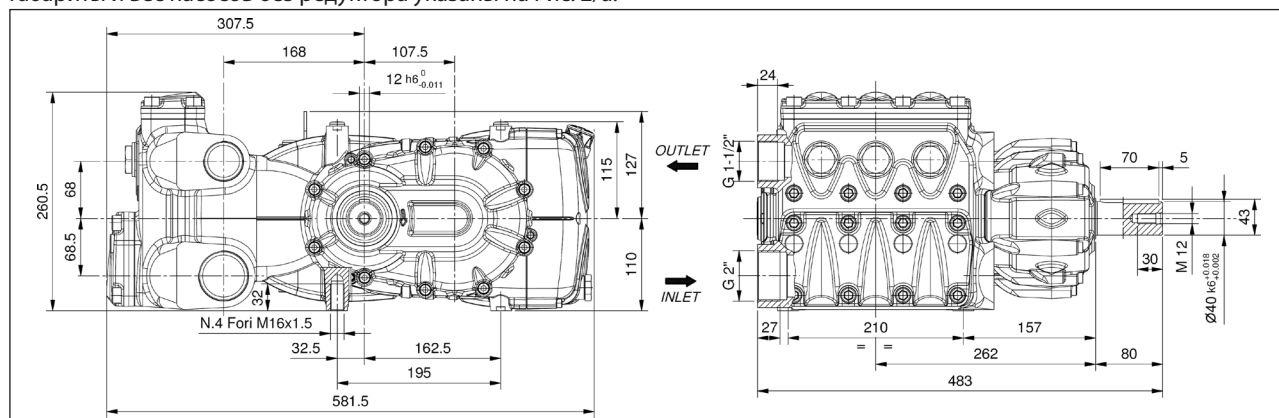
Сухой вес 88 кг
