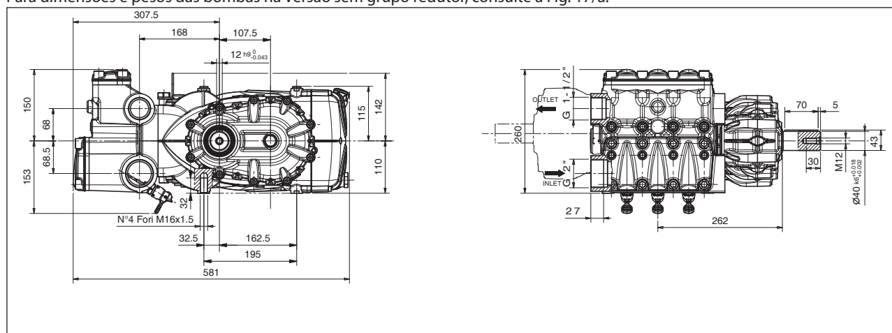
Peso a seco 80 kg.
