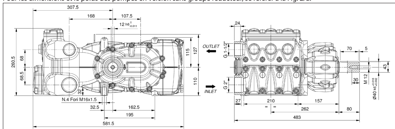
Poids à vide 88 kg.
