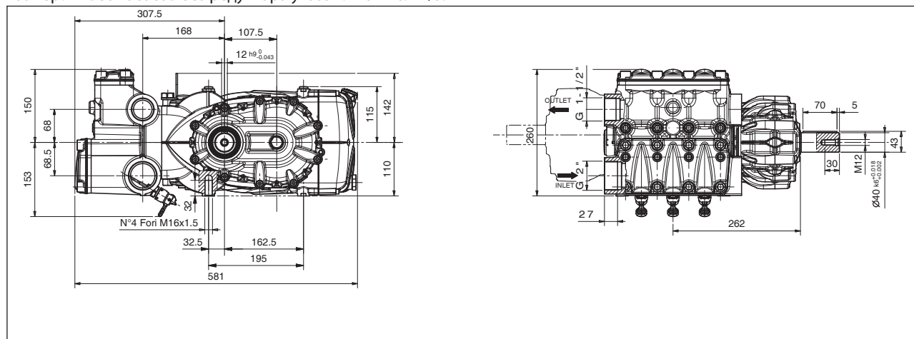
Сухой вес 80 кг
