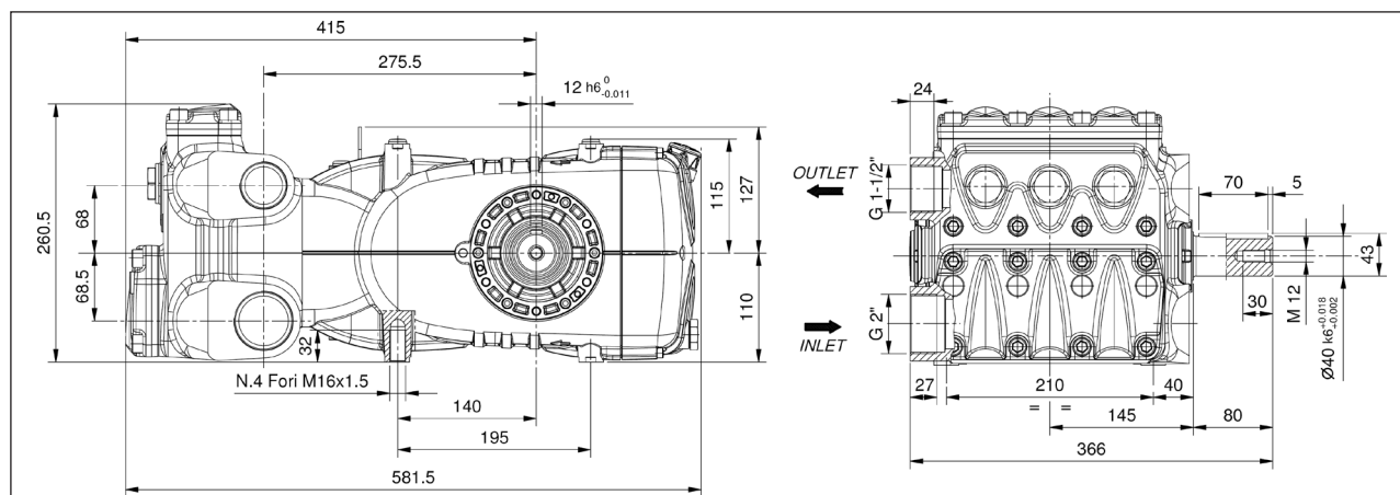
Poids à vide 75 kg.
